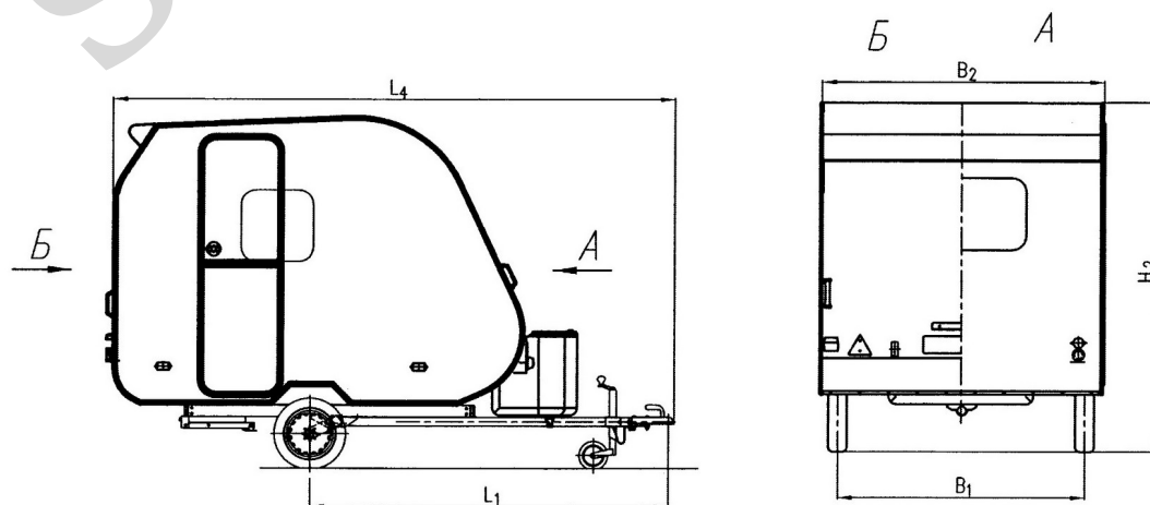
Прицеп «Купава» 811002
