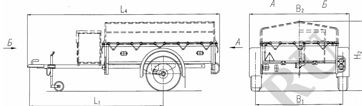
Прицеп «Купава» 811003
