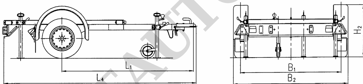
Прицеп «Купава» 811004
