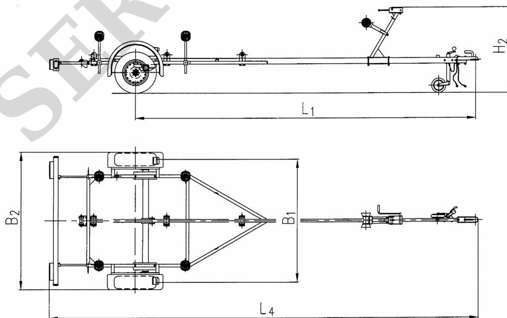
Прицеп «Купава» 811005
