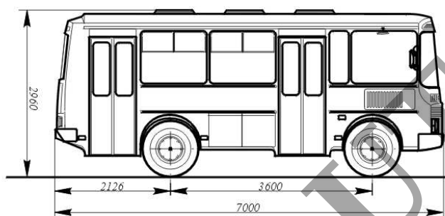
Двухдверная модификация. Вид сбоку
