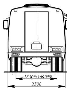
Грузопассажирская модификация. Вид сзади***
