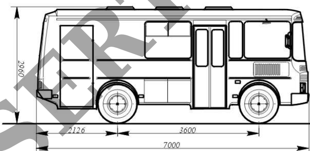
Грузопассажирская модификация. Вид сбоку***
