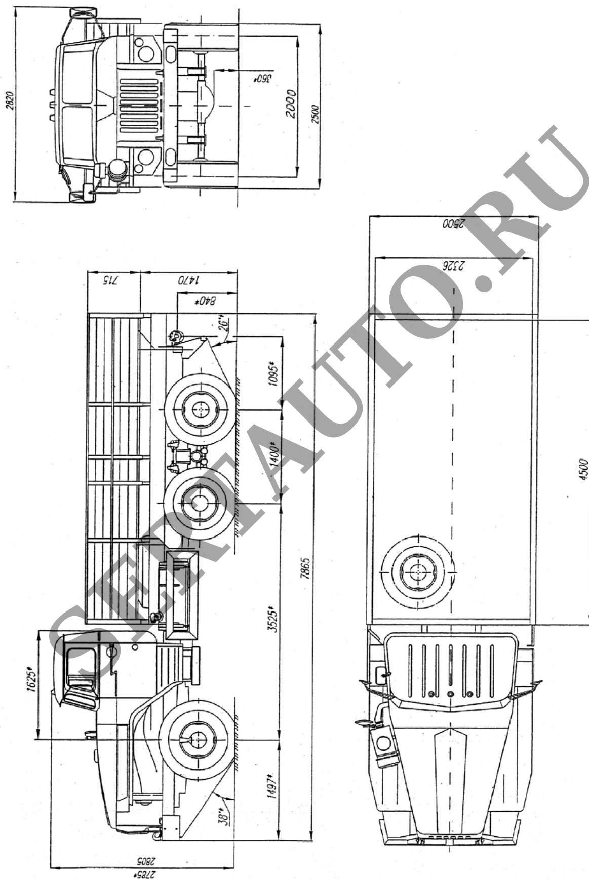
Автомобиль Урал-4320-0611-31
