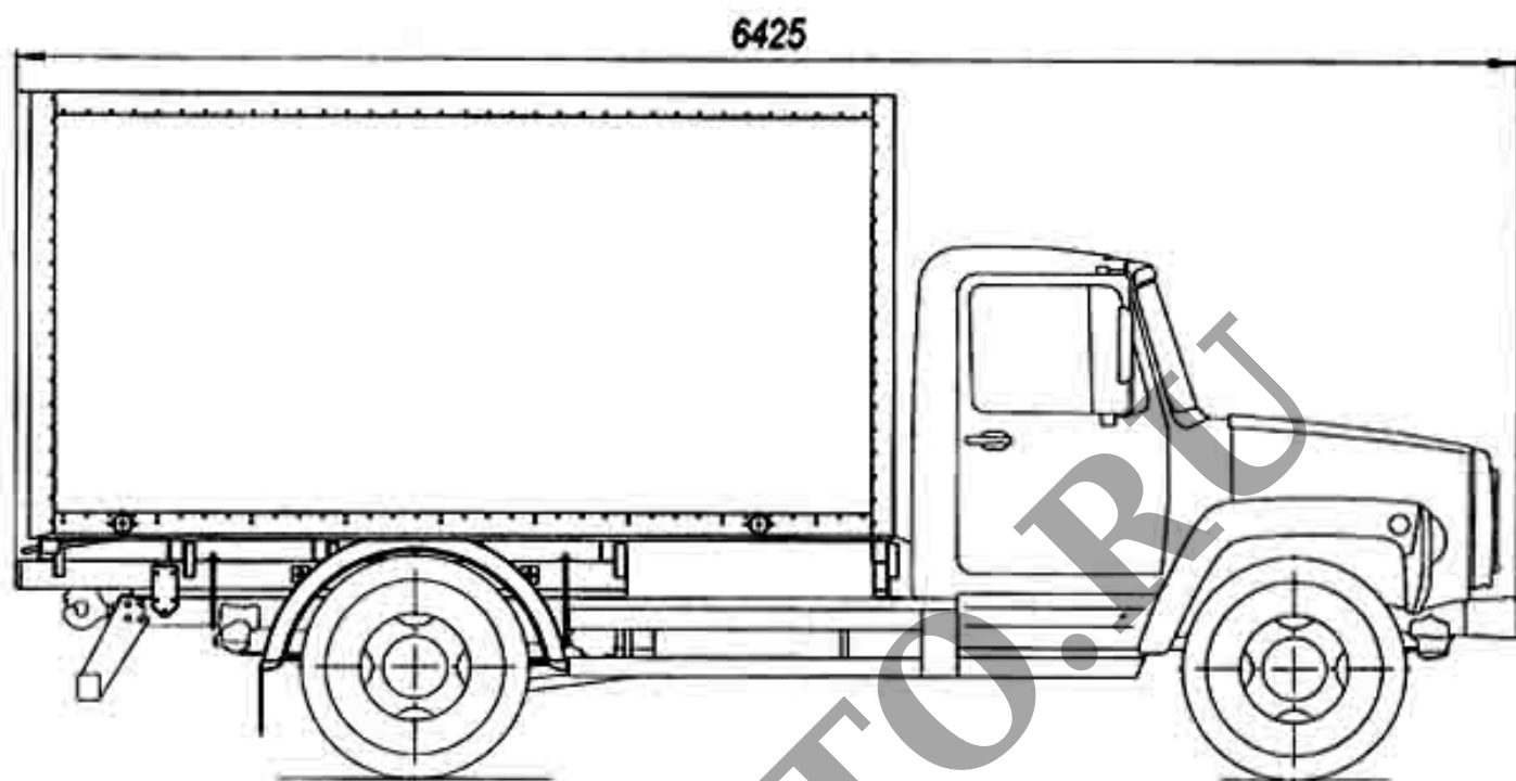
Автомобили-фургоны изотермические на шасси ГАЗ-3307, ГАЗ-3308
