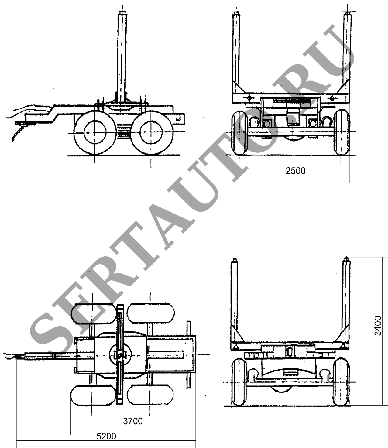
Прицеп-ропуск лесовозный ЛПРУ-05 (9040-0000010)
