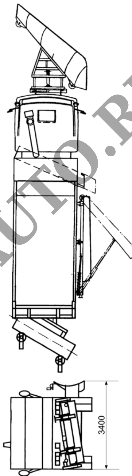
Автомобиль специализированный Машина комбинированная дорожная уборочная 6921ТА (ДМК-40-01) (6921-0000010-06)
