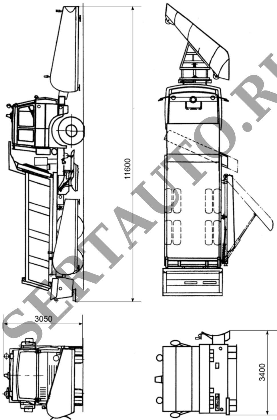
Автомобиль специализированный Машина комбинированная дорожная уборочная 6921T0 (ДМК-40) (6921-0000010-05), 6921ТА (ДМК-40-01) (6921-0000010-06)
