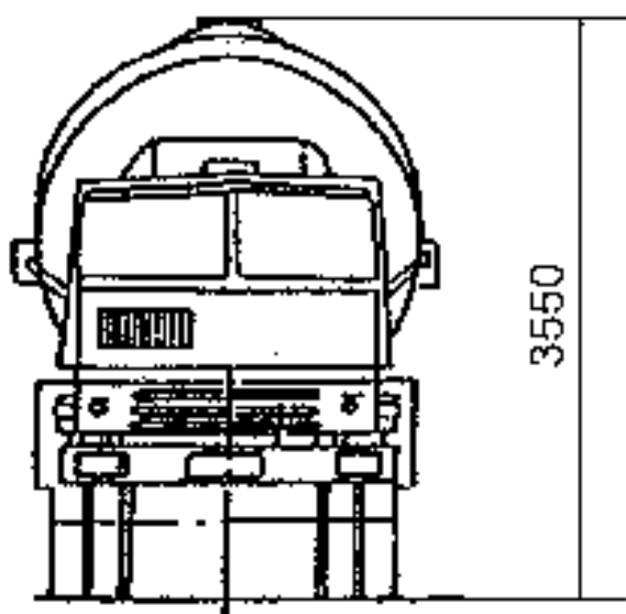
Автобетоносмеситель АБС-6.1-01 (69343-0000010)
