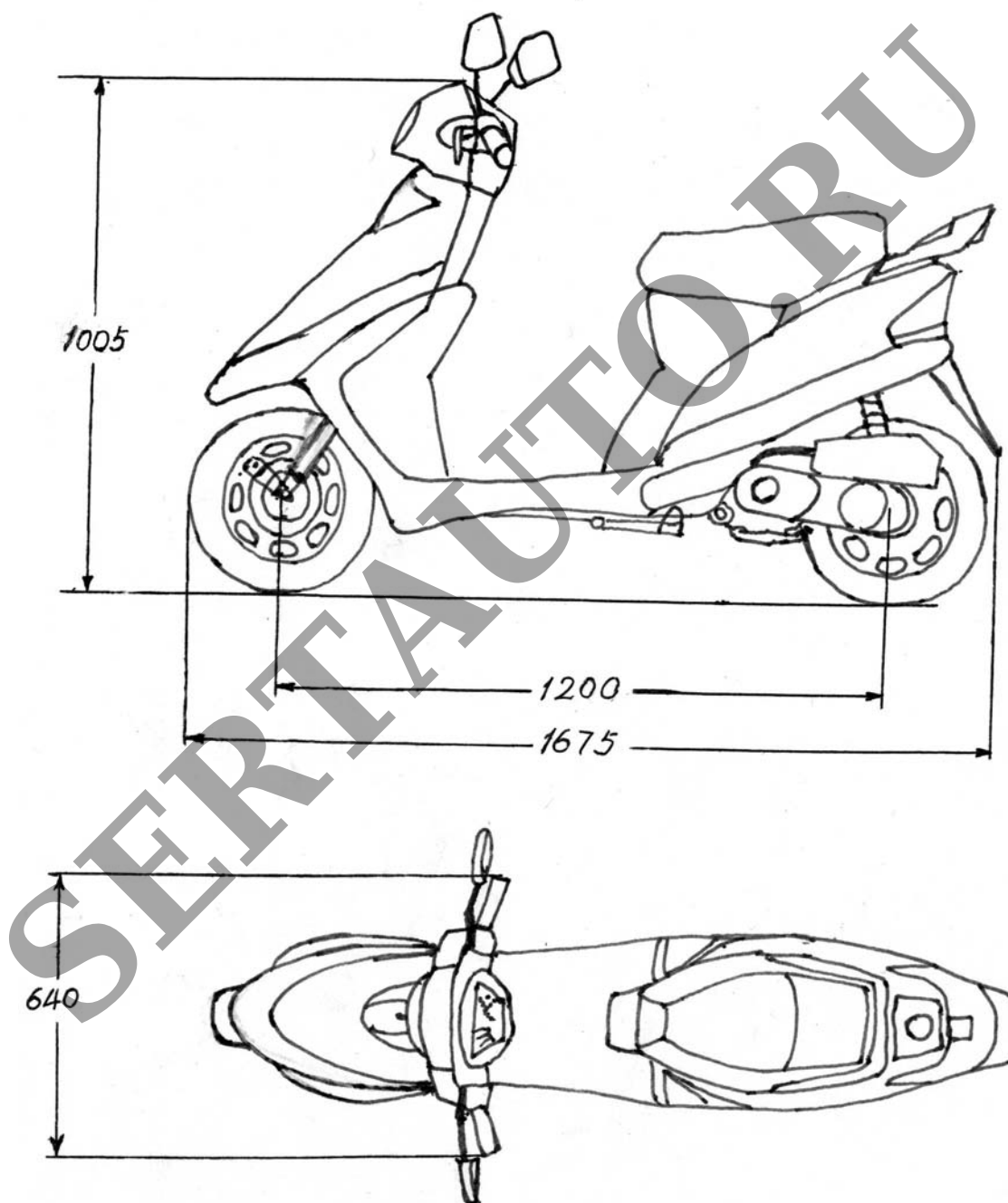
Общий вид мотороллера KINLON модели JL50QT (JL50QT-7A)
