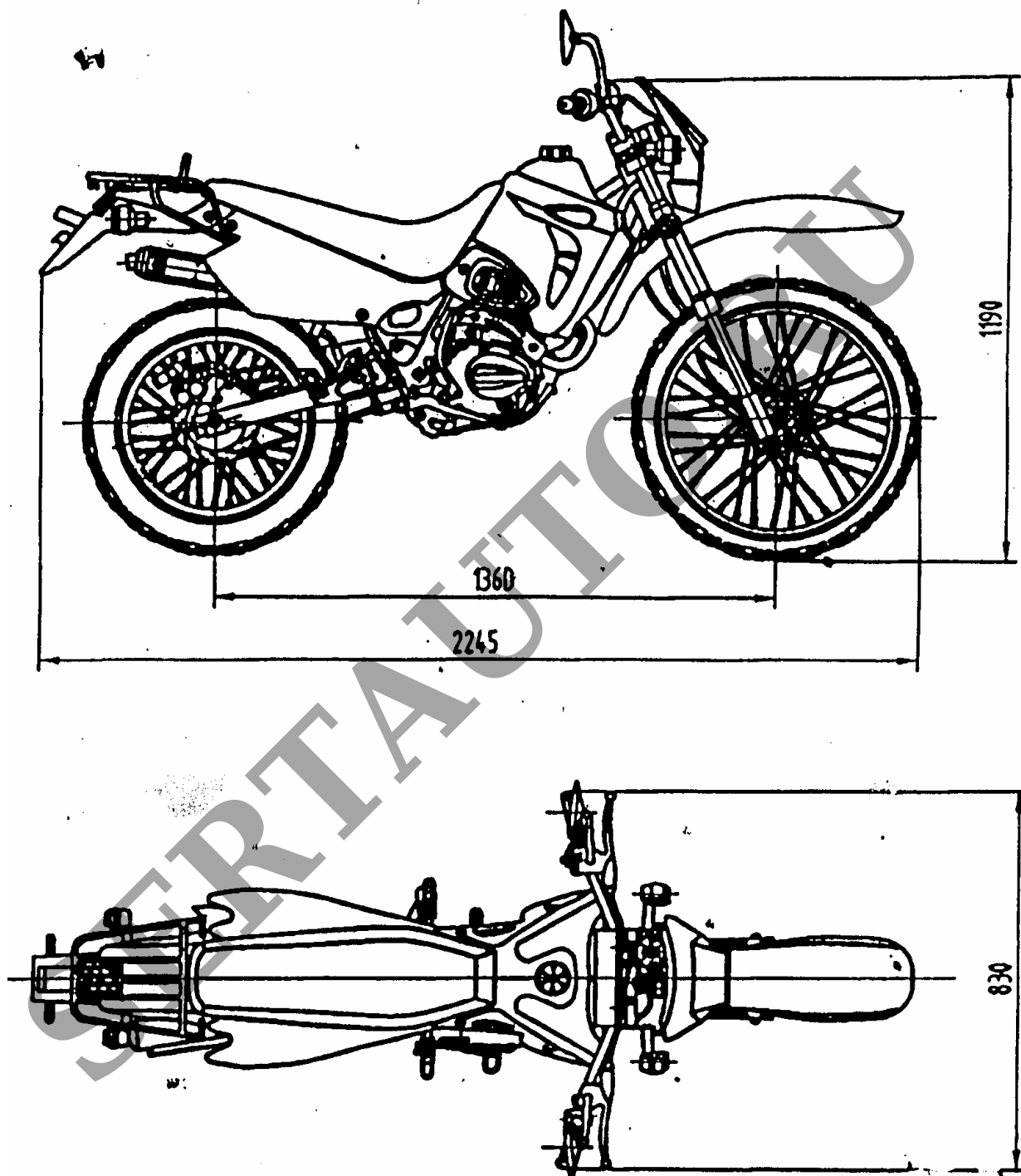
Общий вид мотоцикла SG200GY-2
