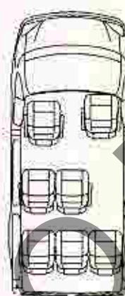
ГАЗ-2217, -22171
