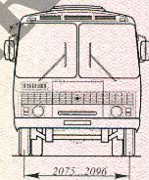
Двухдверная модификация
