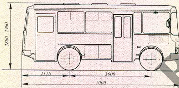
Однодверная модификация
