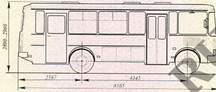
Однодверная модификация
