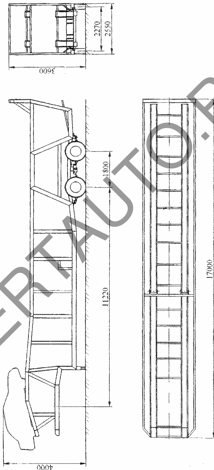
Рис. 1. Полуприцеп - автовоз модели 9963B0
