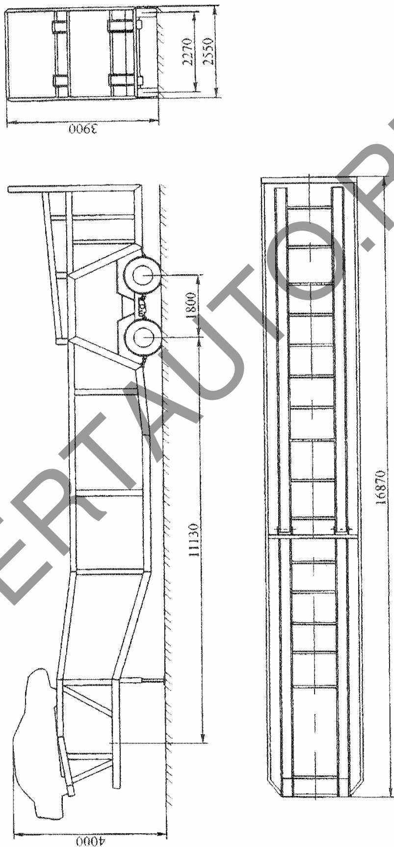
Рис. 1. Полуприцеп - автовоз модели 9963E0
