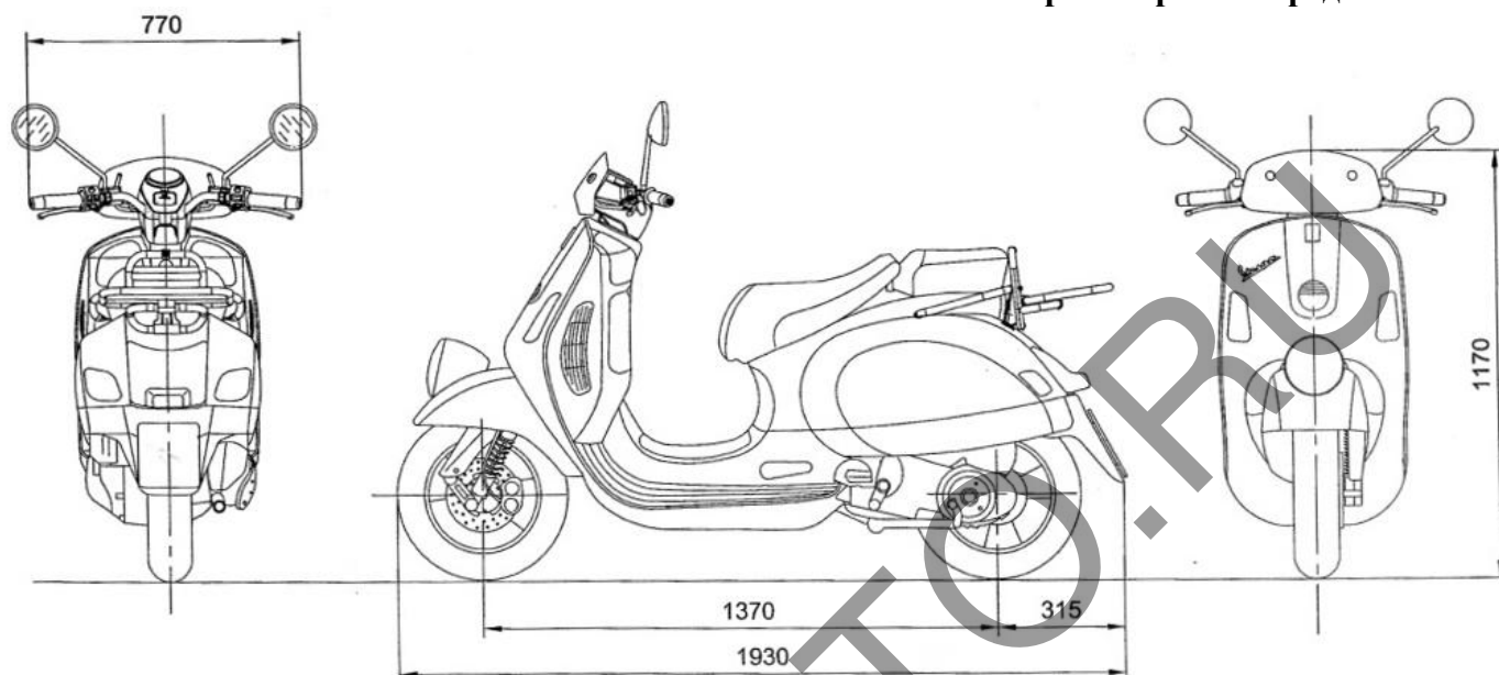
Внешний вид мотоцикла M45 (1/02)
