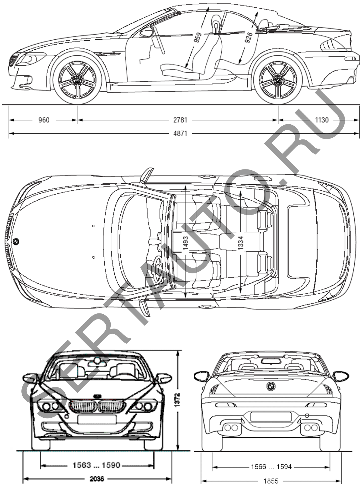
Общий вид автомобиля BMW M560 (M6), кузов «Кабриолет»
