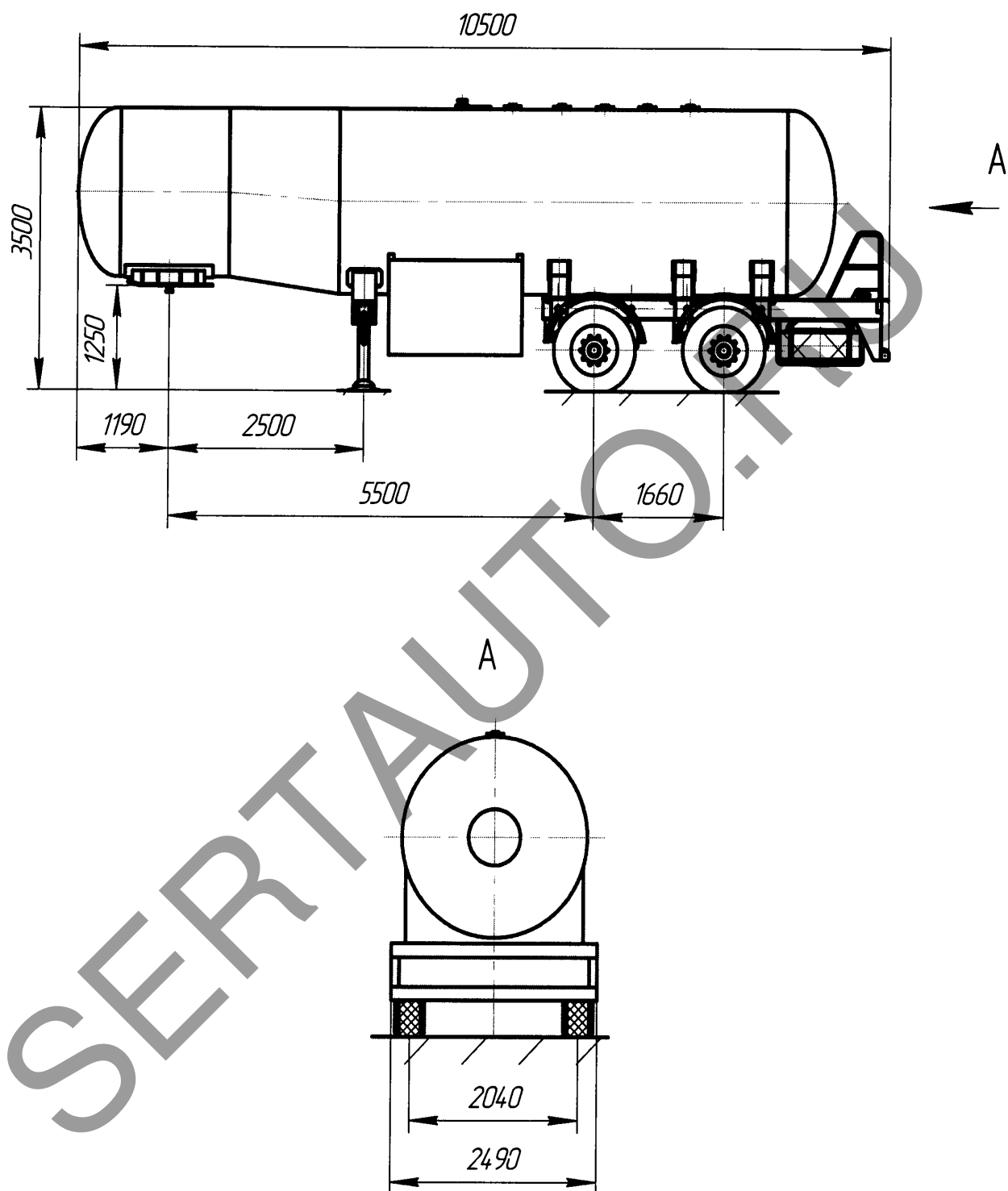
Рис.1. Полуприцеп-цистерна модели 96115-0000010.
