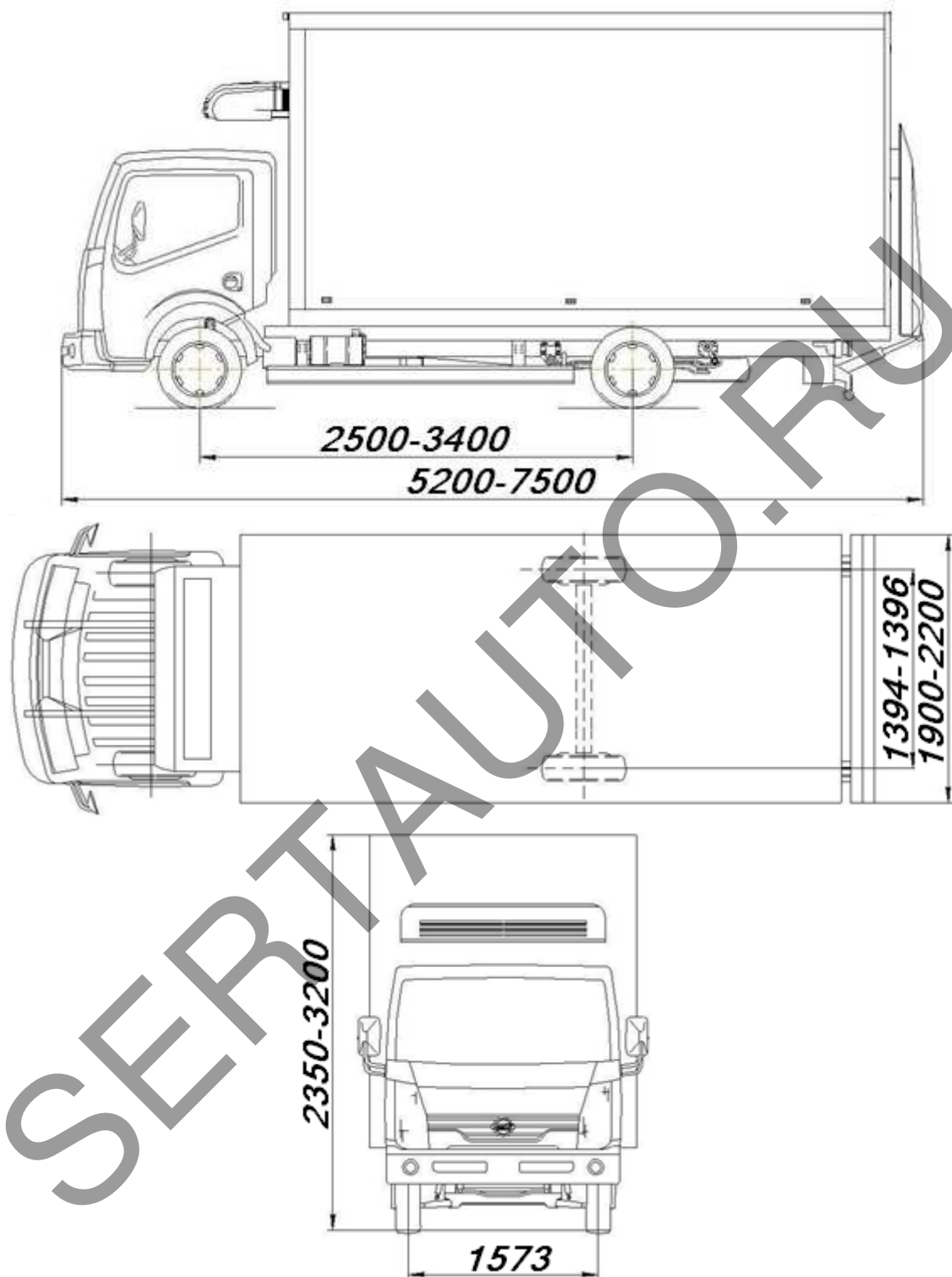
Общий вид автомобиля - фургона рефрижераторного 577882, в исполнении с гидравлическим бортом, на шасси Nissan Cabstar (F 24).
