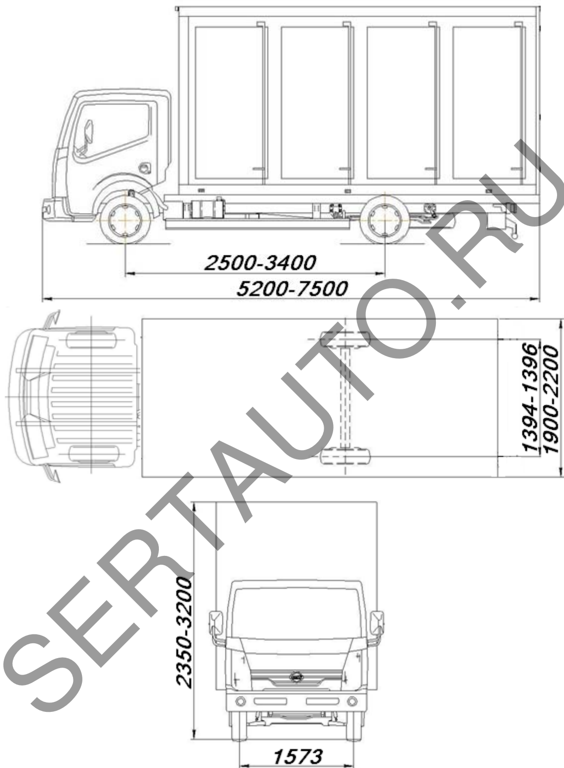
Общий вид автомобиля - фургона хлебного 577885 на шасси Nissan Cabstar (F 24).
