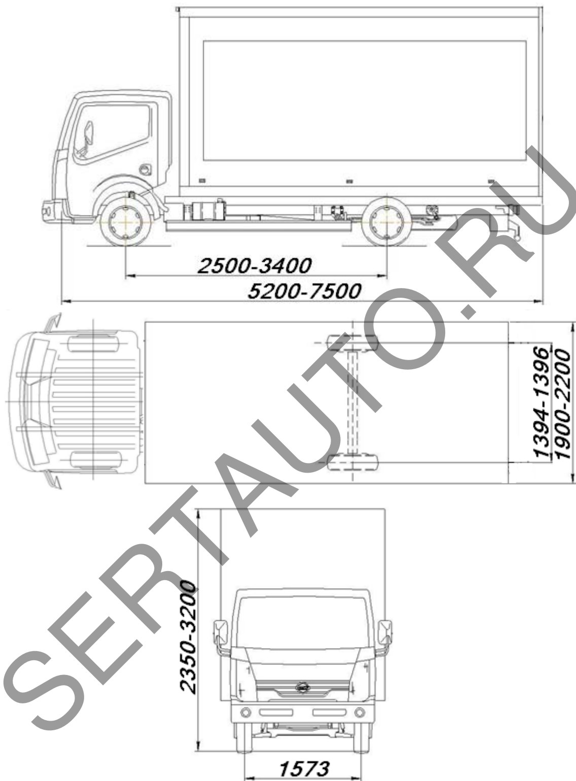
Общий вид автолавки 577888 на шасси Nissan Cabstar (F 24).
