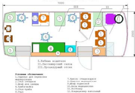
Передвижной медицинский комплекс БМК-3033-011-14 "Кабинет семейного врача - Семейный доктор" на базе автобуса ПАЗ-3205
