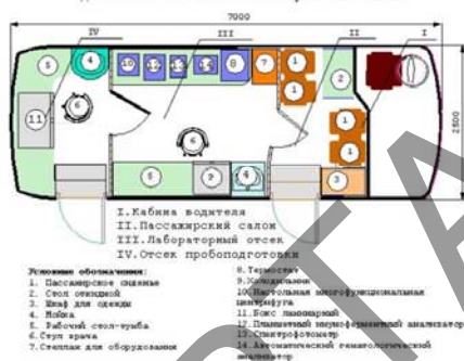
Передвижной лабораторный комплекс ВМК-3033-210-05 "Лаборатория ветеринарного надзора - Комплексная диагностика" на базе автобуса ПА3-32053
