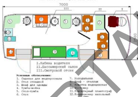
Передвижной медицинский комплекс ВМК-3033-013-09 "Диагностический кабинет - "Здоровый ребенок" на базе автобуса ПАЗ-3205
