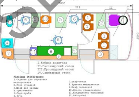
Передвижной медицинский комплекс ВМК-3033-015-09 "Диагностический кабинет - Диагностика сахарного диабета" на базе автобуса ПАЗ-3205
