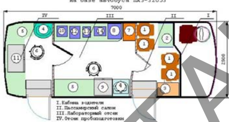
Передвижной лабораторный комплекс БМК-3033-010-05 "Комплексная диагностическая лаборатория" на базе автобуса ПАЗ-32053
