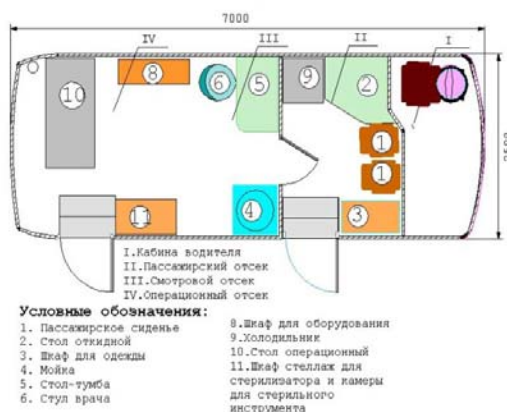
Передвижной ветеринарный комплекс ВМК-3033-26 "Скорая ветеринарная помощь" на базе автобуса ПАЗ-3205
