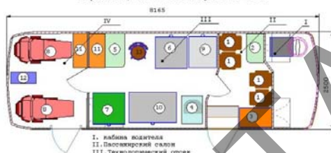
Передвижной медицинский комплекс БМК-30331-011-06 "Донор" (Донация, переработка, хранение, транспортировка донорской крови. Вариант 2) на базе автобуса ПАЗ-4234
