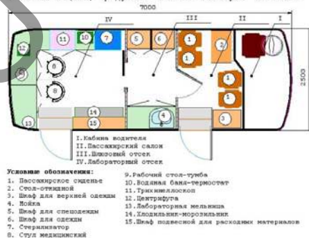
Передвижной лабораторный комплекс БМК-3033-115-05 "Санитарно-эпидемиологическая лаборатория - Экспертиза качества пищевых продуктов" на базе автобуса ПАЗ-3205
