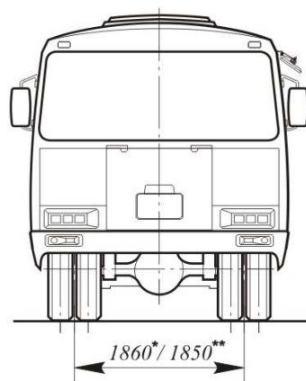
Вид сзади
