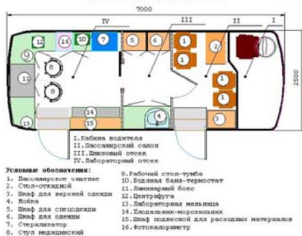
Передвижной лабораторный комплекс ВМК-3033-118-05 "Санитарно-эпидемиологическая лаборатория - Токсикологическая" на базе автобуса ПА3-3205
