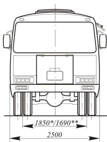
Вид сзади
