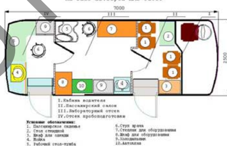
Передвижной лабораторный комплекс ВМК-3033-212-05 "Лаборатория ветеринарного надзора - ИФА-лаборатория" на базе автобуса ПА3-32053
