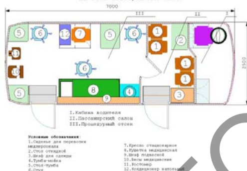
Передвижной медицинский комплекс ВМК-3033-011-14 "Кабинет семейного врача - Семейный доктор" на базе автобуса ПАЗ-3205
