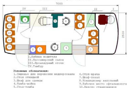
Передвижной медицинский комплекс ВМК-3033-011-09 "Диагностический кабинет - Диагностика глазных болезней" на базе автобуса ПАЗ-3205
