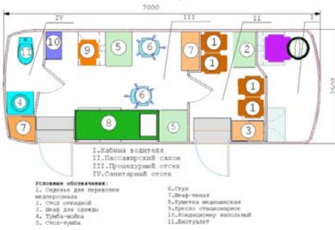
Передвижной медицинский комплекс ВМК-3033-016-09 "Диагностический кабинет - Компьютерная диагностика" на базе автобуса ПАЗ-3205
