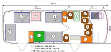
Передвижной медицинский комплекс БМК-30331-030-06 "Донор" (Переработка, хранение, транспортировка донорской крови) на базе автобуса ПАЗ-4234
