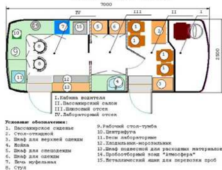
Передвижной лабораторный комплекс БМК-3033-117-05 "Санитарно-эпидемиологическая лаборатория - Радиологическая" на базе автобуса ПАЗ-3205
