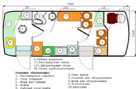
Передвижной лабораторный комплекс БМК-3033-112-05 "Санитарно-эпидемиологическая лаборатория - ИФА-лаборатория" на базе автобуса ПАЗ-32053
