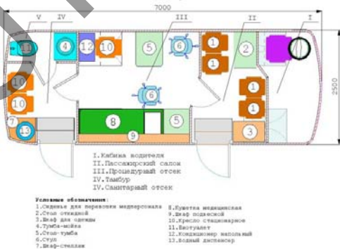
Передвижной медицинский комплекс ВМК-3033-014-09 "Диагностический кабинет - функциональная диагностика" на базе автобуса ПАЗ-3205
