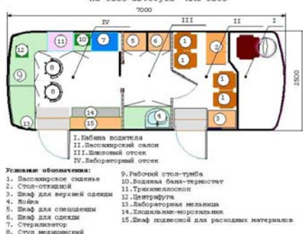
Передвижной лабораторный комплекс ВМК-3033-215-05 "Лаборатория ветеринарного надзора - Экспертиза качества пищевых продуктов" на базе автобуса ПАЗ-3205
