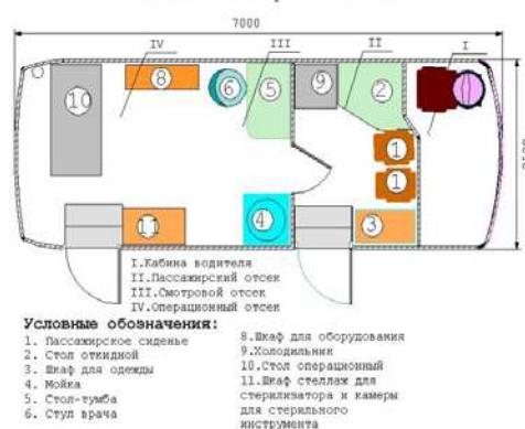
Передвижной ветеринарный комплекс БМК-3033-26 "Скорая ветеринарная помощь" на базе автобуса ПАЗ-3205
