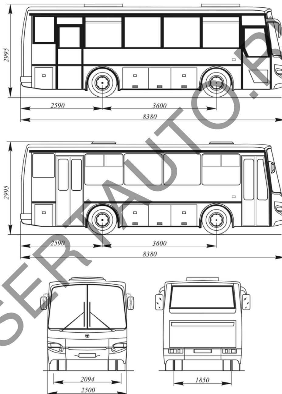
Общий вид автобуса ПАЗ типа 4230??-03
