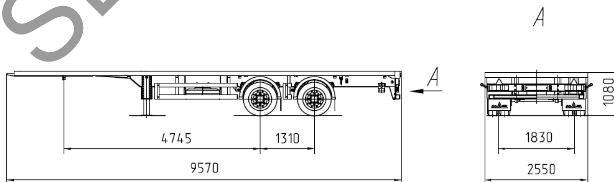
Рис. 3. Полуприцеп МАЗ-931020 (платформа без бортов)
