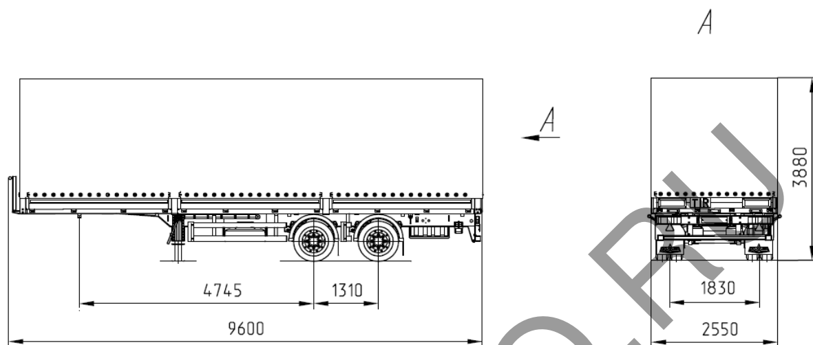
Рис. 1. Полуприцеп МАЗ-931020 (бортовая платформа с тентом)
