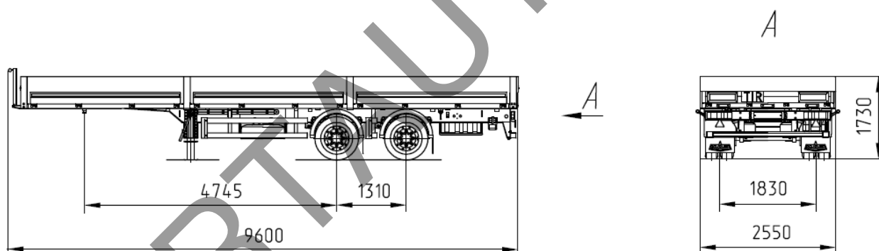
Рис. 2. Полуприцеп МАЗ-931020 (бортовая платформа без тента)
