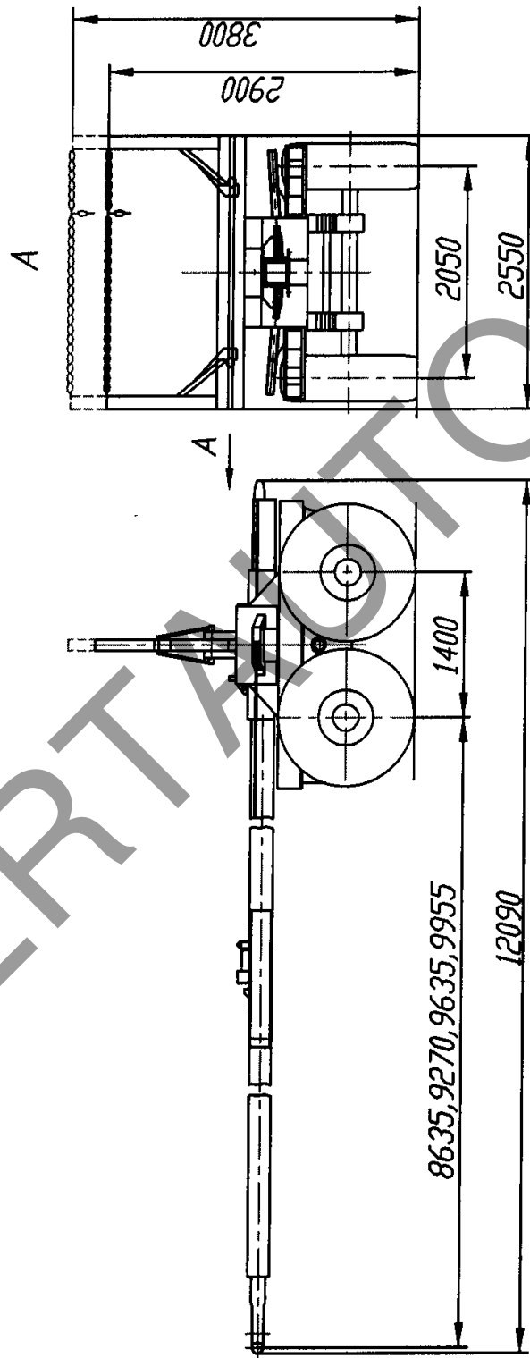
Рис. 3. Прицеп модели МАЗ 900810 (односкатная ошиновка)
