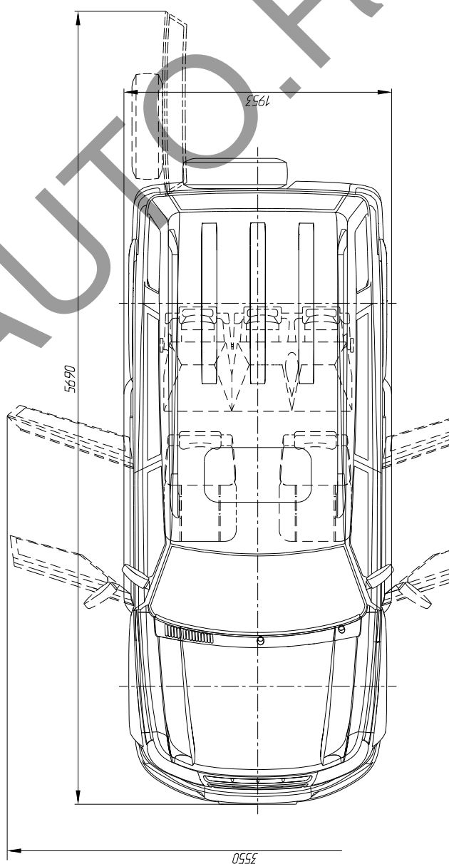
Общий вид УАЗ-3163, УАЗ-31631, 31638 (УАЗ Патриот / UAZ Patriot) с багажными дугами
