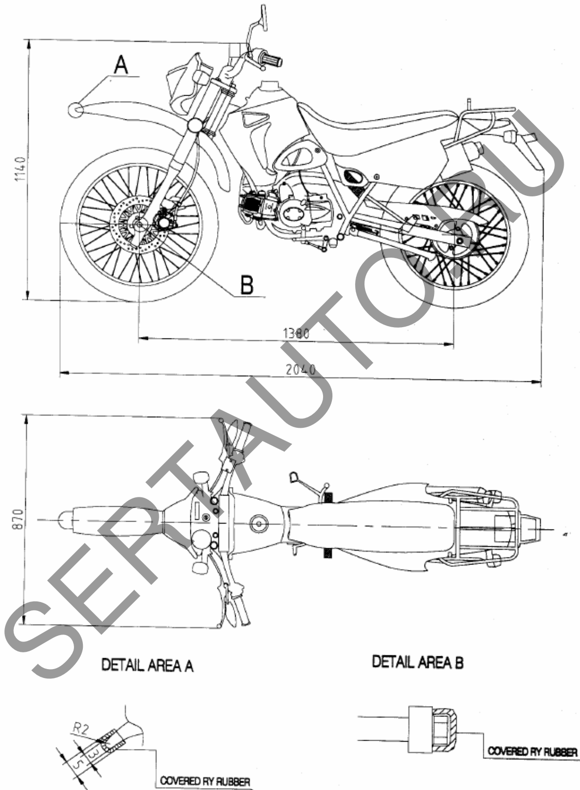
Рис. 1. Мопед YAMASAKI, MINBAN: YM50GYS.
