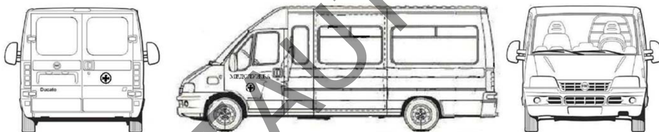
Общий вид цветографической схемы автомобиля медицинской службы
