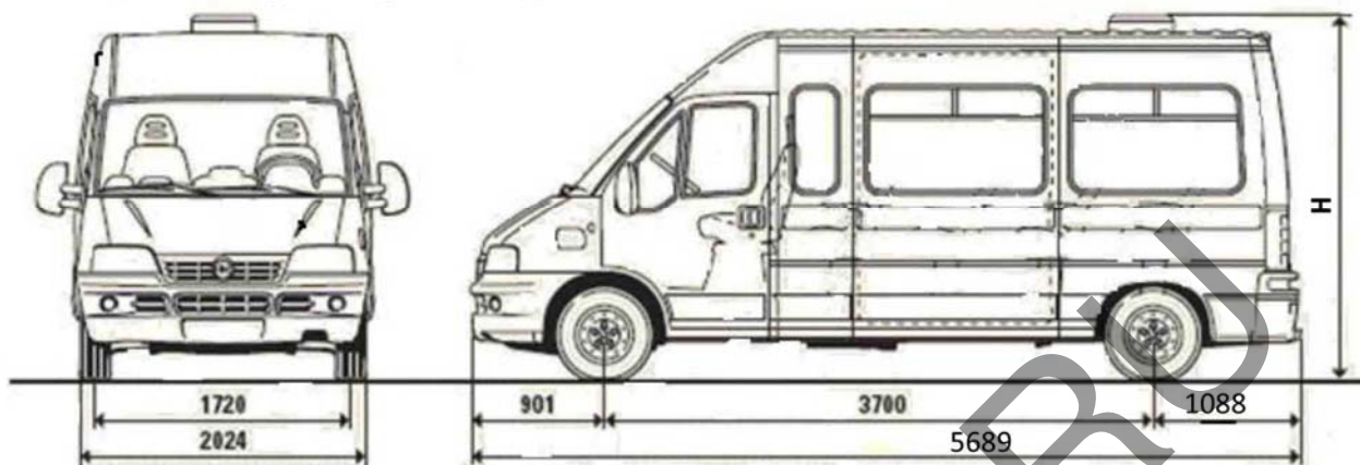
Общий вид транспортного средства FIAT 244 CSMMC-RT, 244 CSWMC-RT
