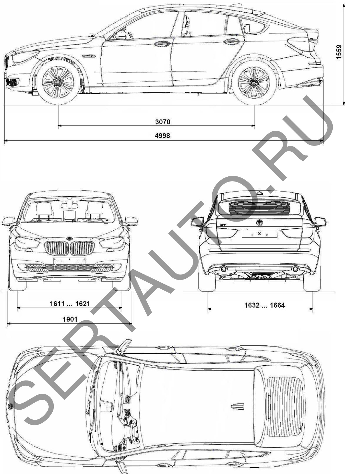
Общий вид автомобилей BMW тип GT
