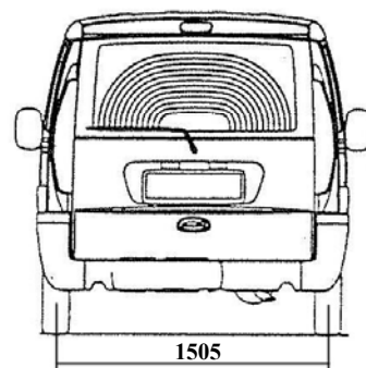
Вариант 1 исполнения задней двери
