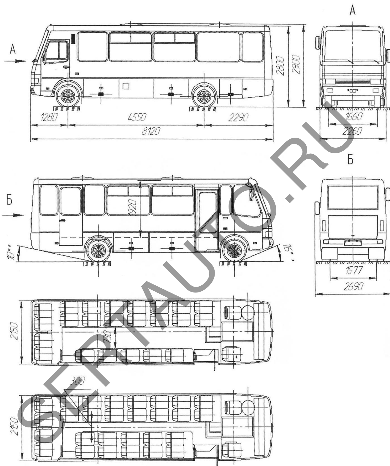
Автобус БАЗ-А079.34
