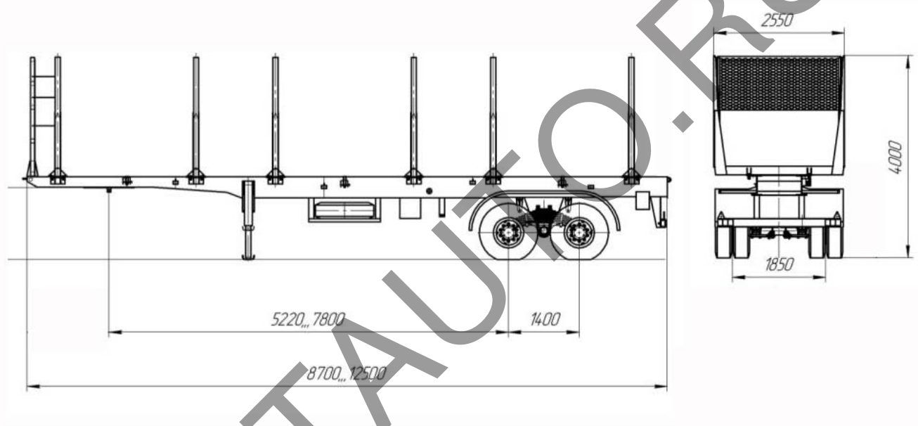
Общий вид полуприцепа-сортиментовоза 844602
