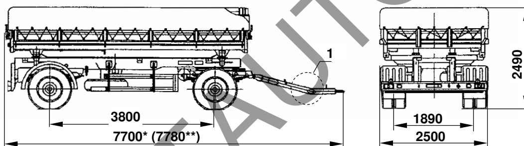
металлическая самосвальная платформа с откидными боковыми бортами и с дополнительными деревянными бортами и тентом
