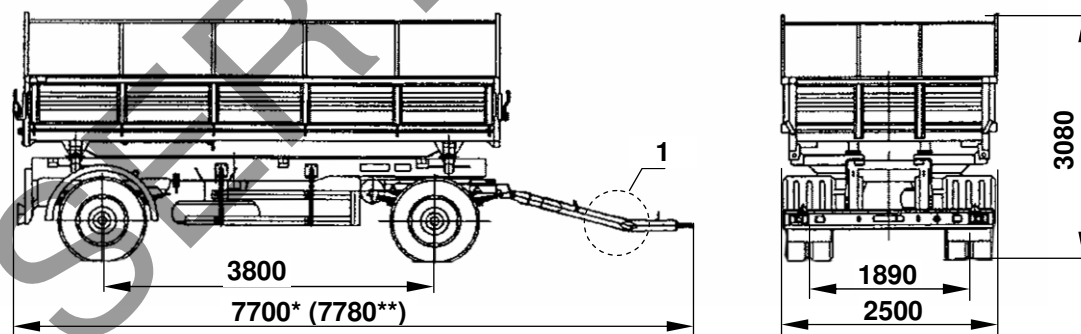
металлическая самосвальная платформа с откидными боковыми бортами и надставными металлическими бортами
