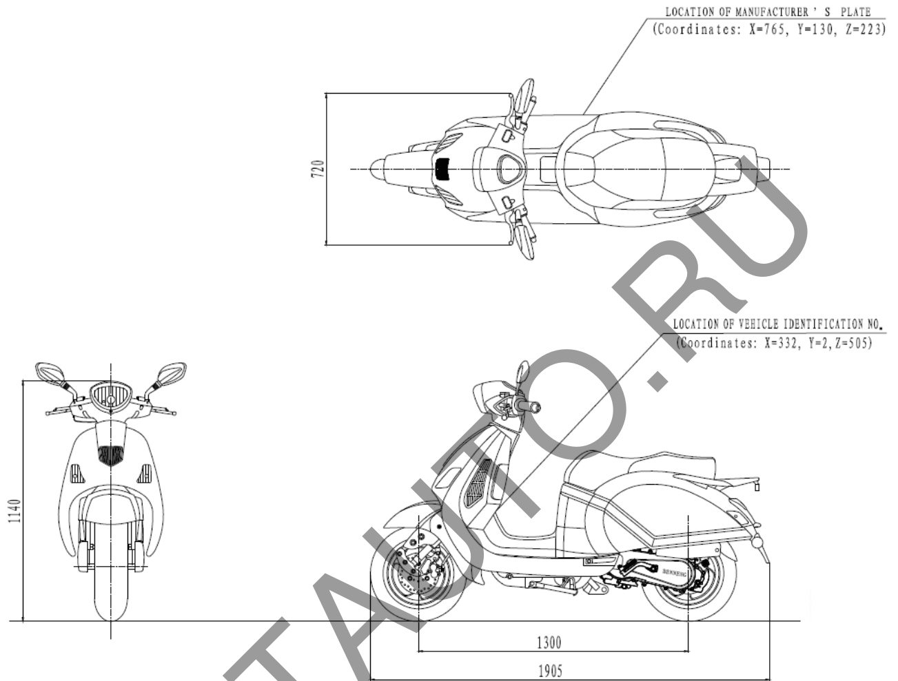
Рис. 1. Мотоцикл ZNEN, ZN125T-F.
