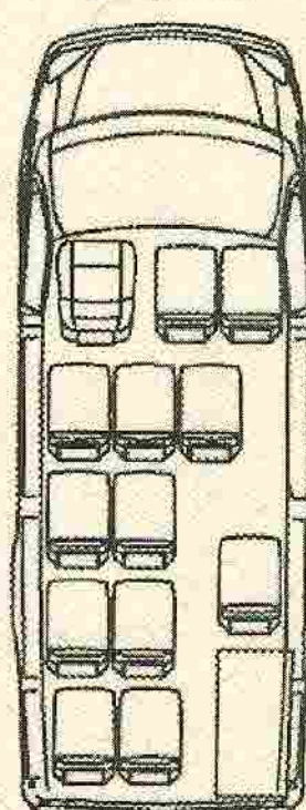
ГАЗ-322121, -322171
