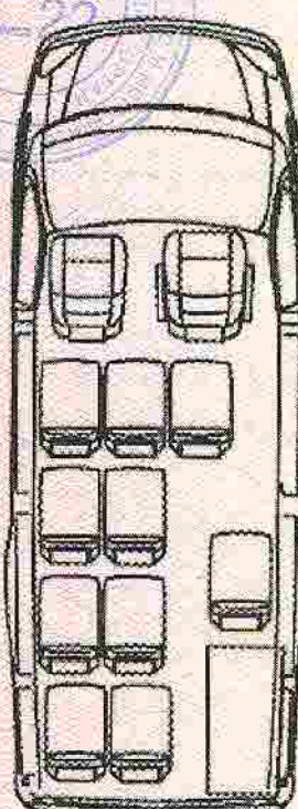
ГАЗ-322121, -322171
