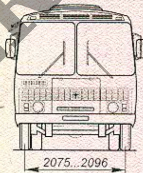
Двухдверная модификация
