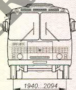
Двухдверная модификация
