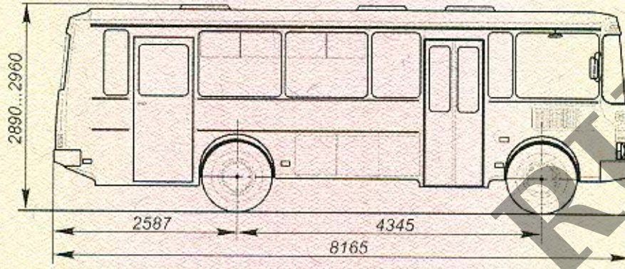
Одностворная модификация
