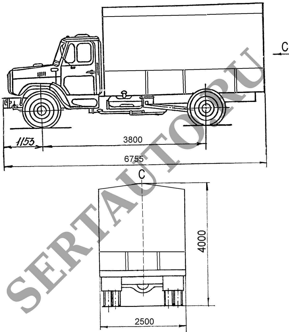
Рис. 4. Автомобиль с бортовой платформой и тентом модели 47440Н на шасси (базе) ЗИЛ 432930, ЗИЛ 432932
