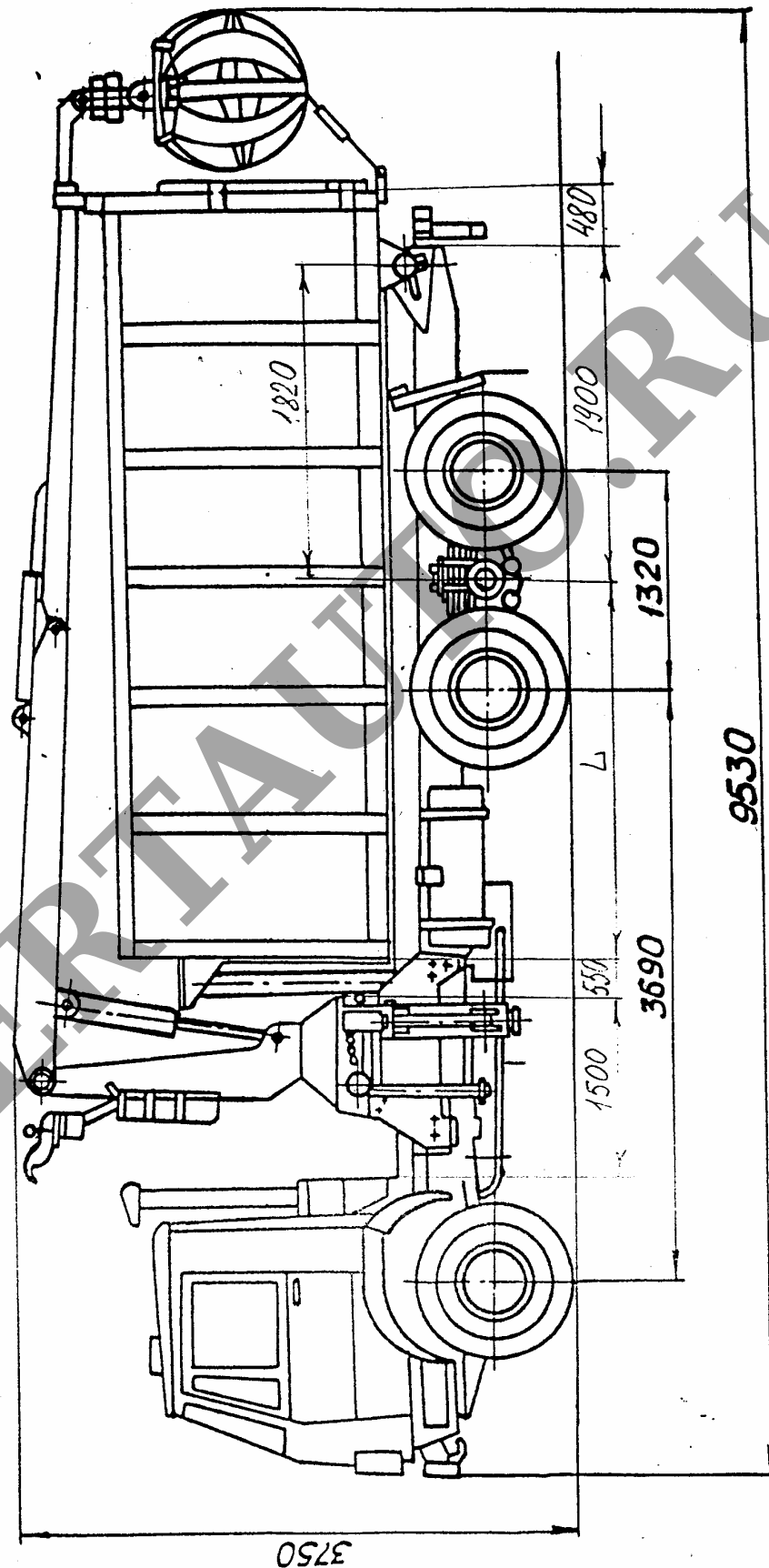
Рис. 1. Автомобиль самосвал с краном манипулятором моделей: 581100 (5811-0000010-01), 58110А (5811-0000010-02)
