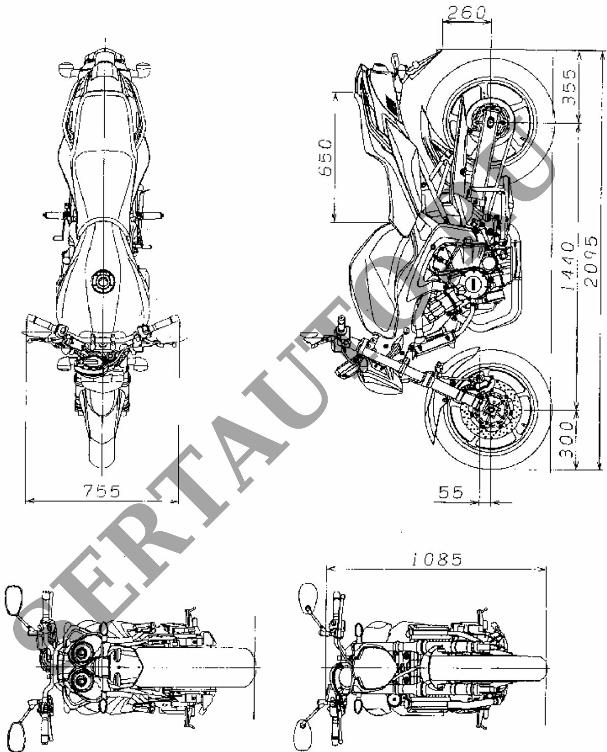
Рис.5. Мотоцикл YAMAHA RJ07 (FZS 600N) вариант исполнения II/v, II/vi, II/vii
