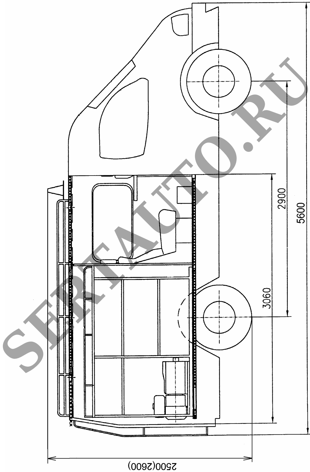
Рис. 1. Автомобиль - мастерская модели 29620L (2962-000010-31) / МММ (машина мостового мастера)
