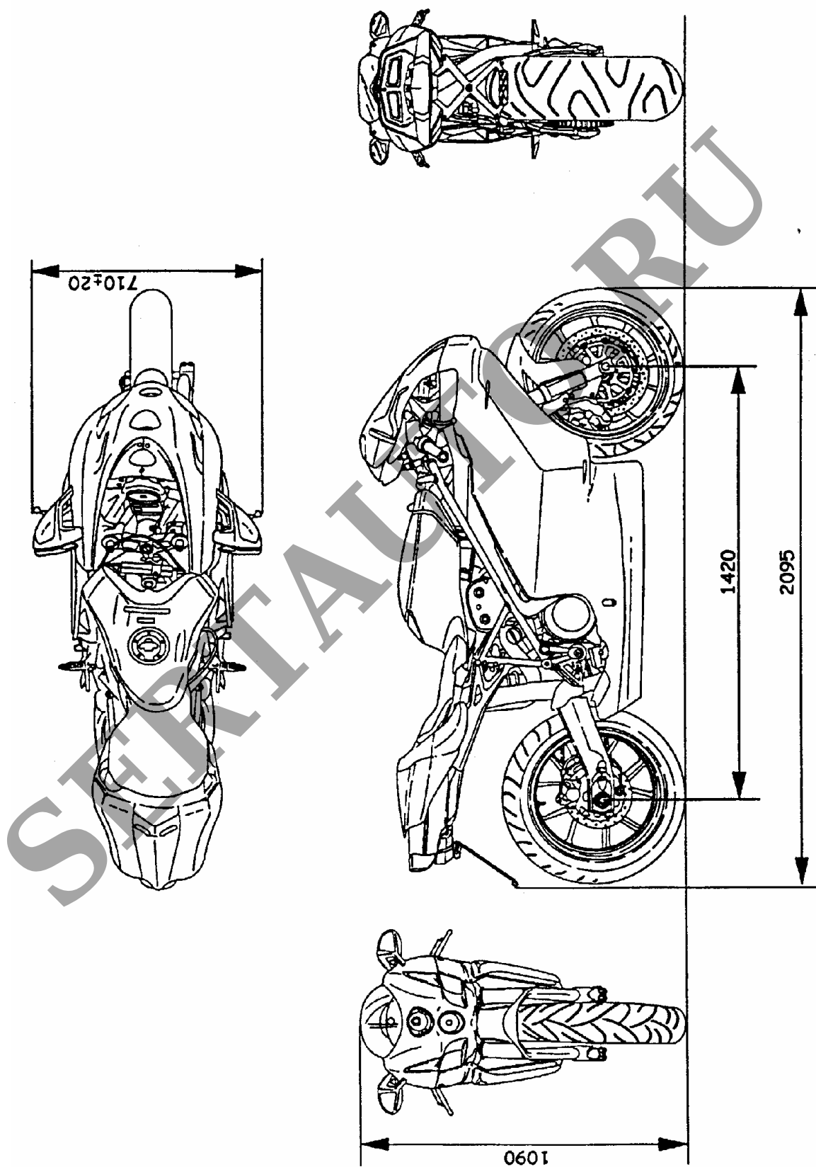
Рис. 4. Мотоцикл DUCATI SUPERBIKE моделей 999 (H4), 999S (H4).
