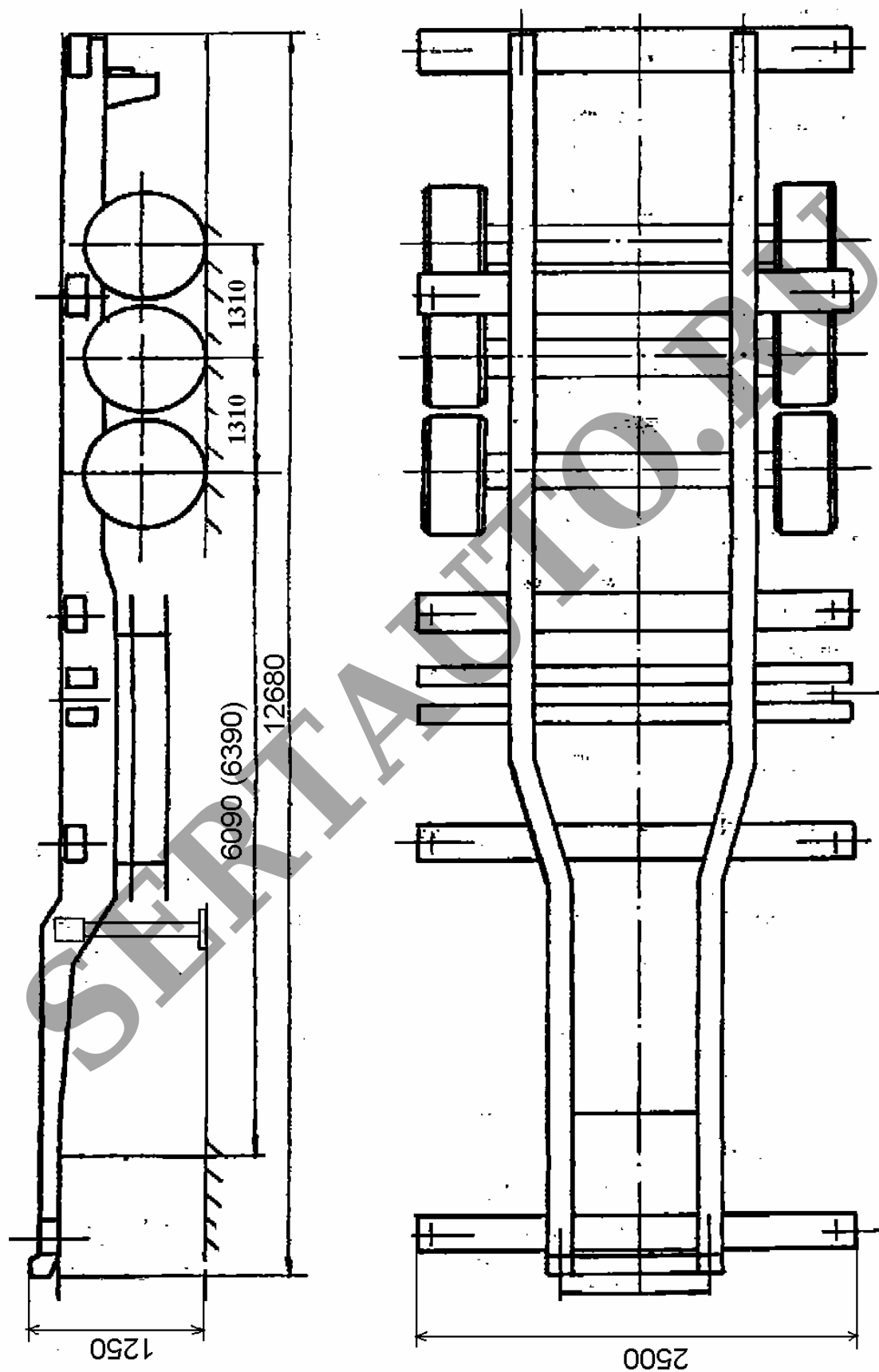
Рис.2. Полуприцеп контейнеровоз модели SCF 24 G
