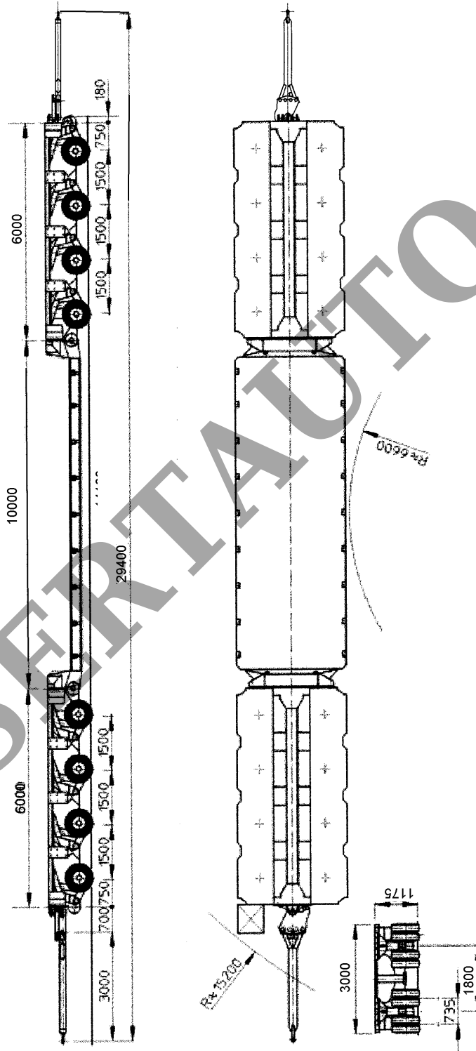
Рис.3. Прицеп GOLDHOFER модели THP / SL , версия 21 , с двумя модулями THP / SL 4
