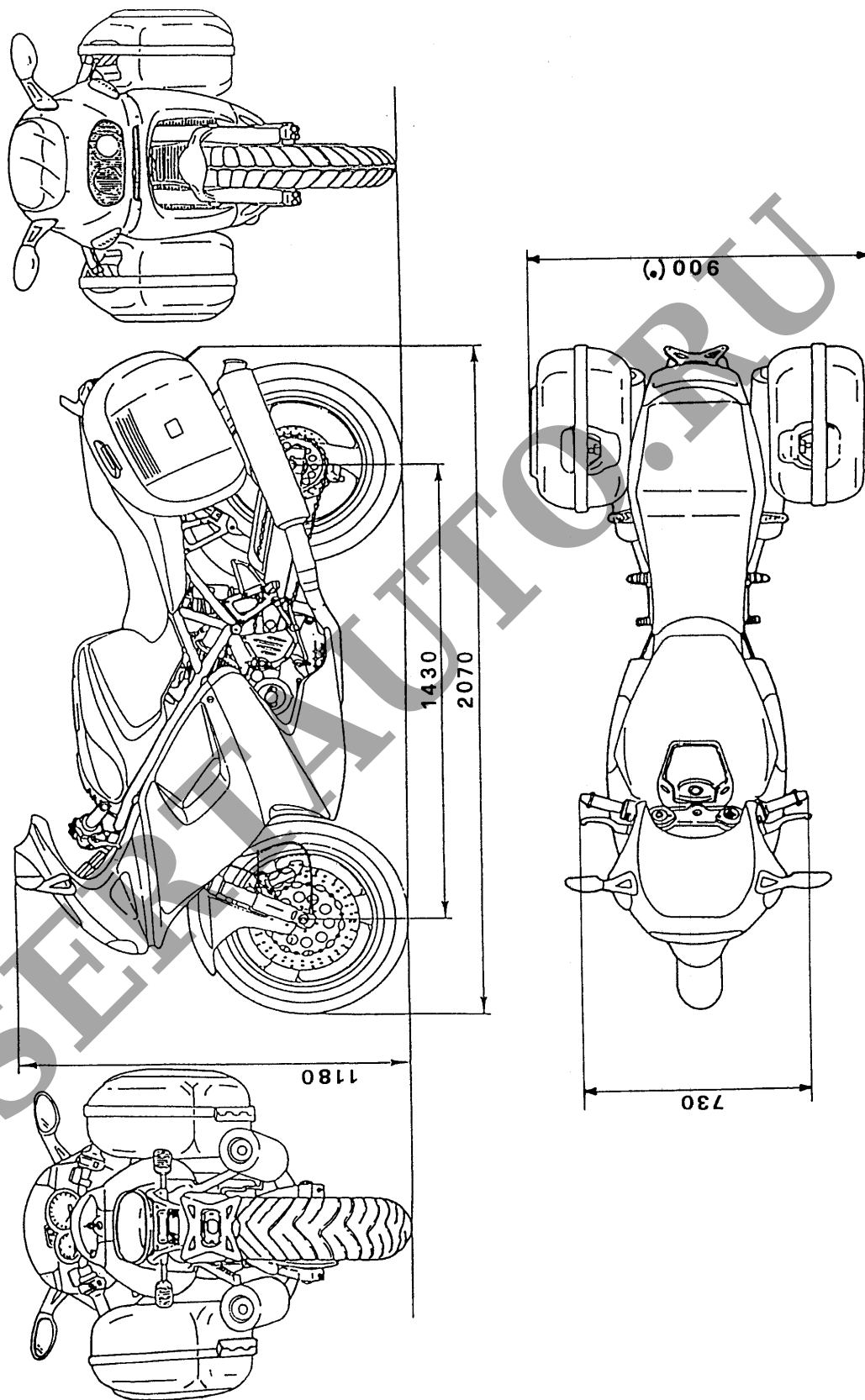
Рис. 2. Мотоцикл DUCATI SPORT TOURING (S1,S2) моделей: ST 2, ST 4, ST 4S, ST 4S-ABS с боковыми кофрами
