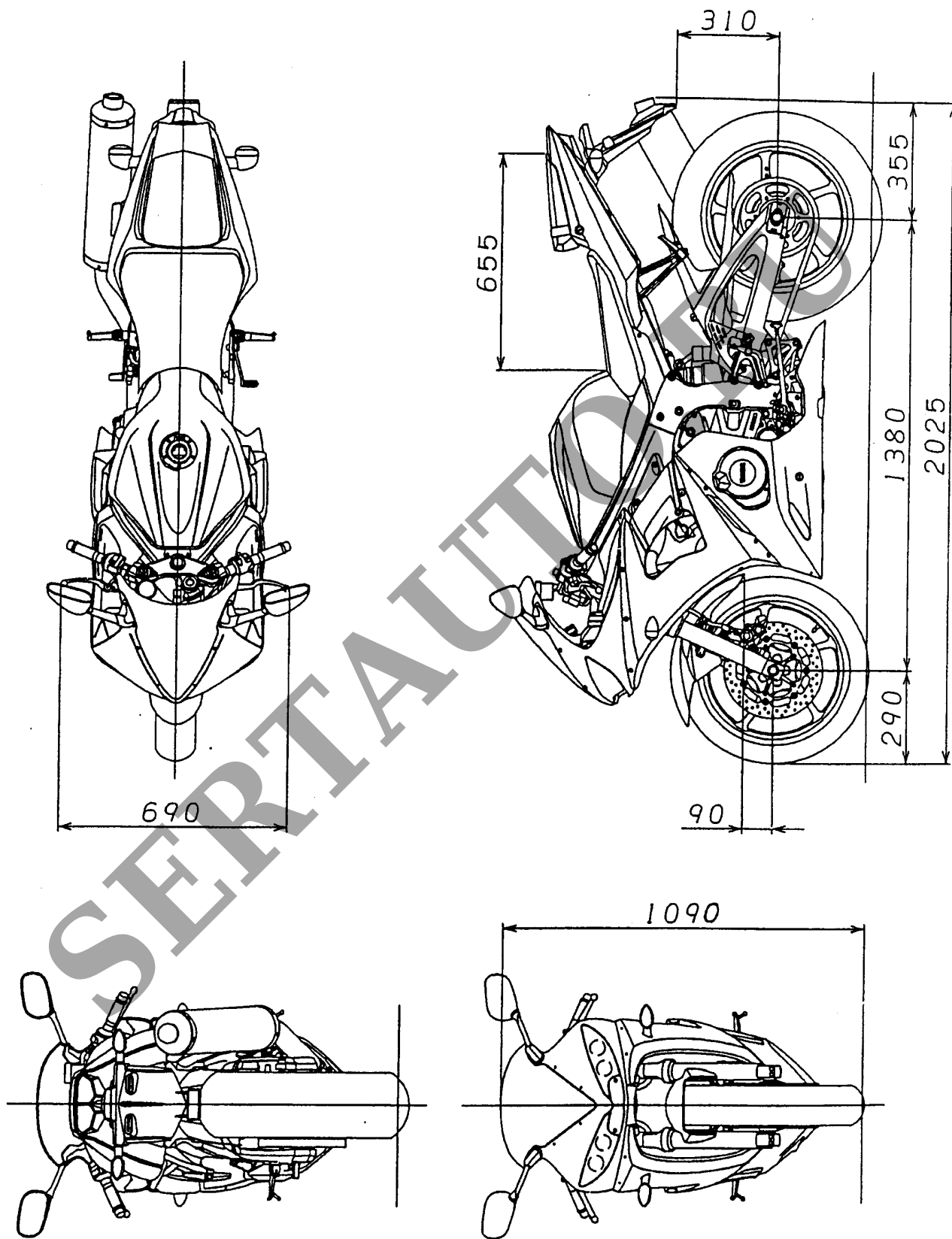
Рис. 1. Мотоцикл YAMAHA модели YZF-R6 тип RJ05.
