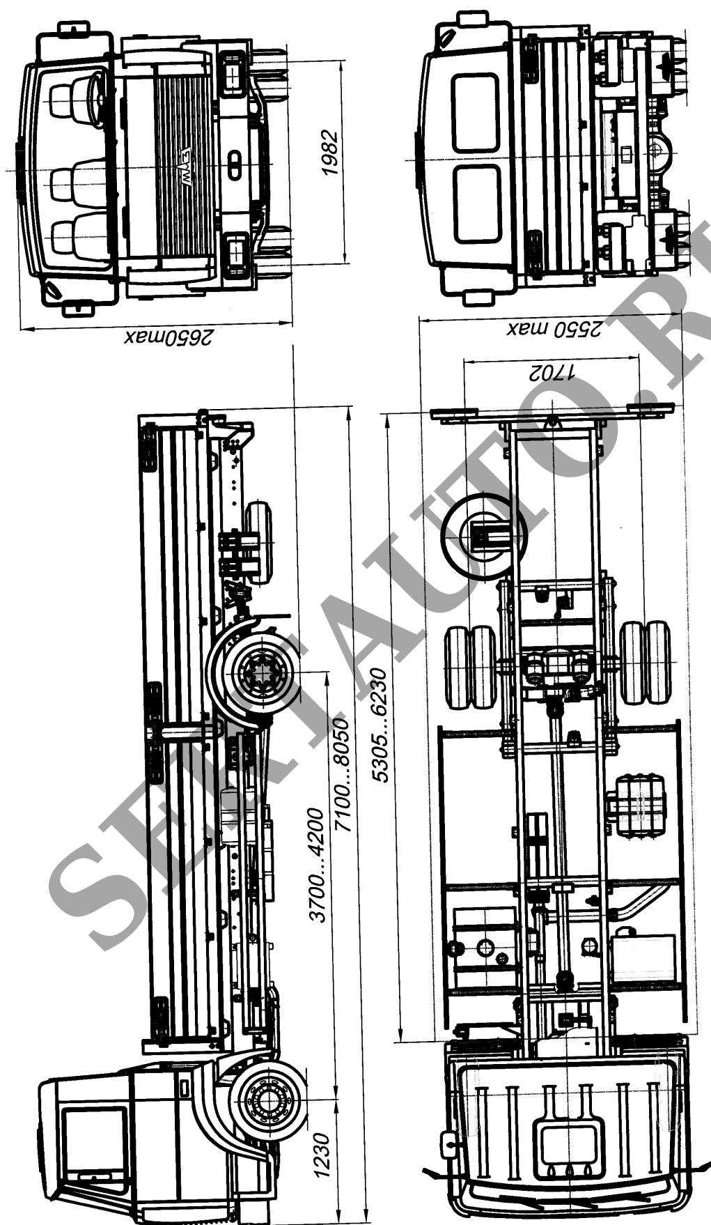
Рис.3 Автомобиль МАЗ 437040 с бортовой платформой
