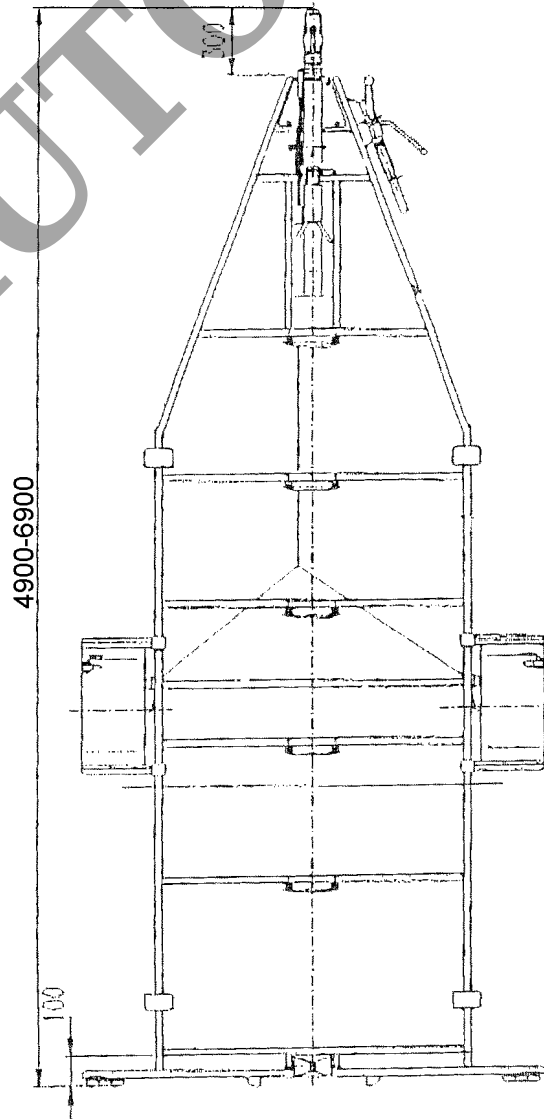
Рис. 1 Прицеп к легковым автомобилям моделей: PC 1000..., PC 1100..., PC 1200..., PC 1500...
