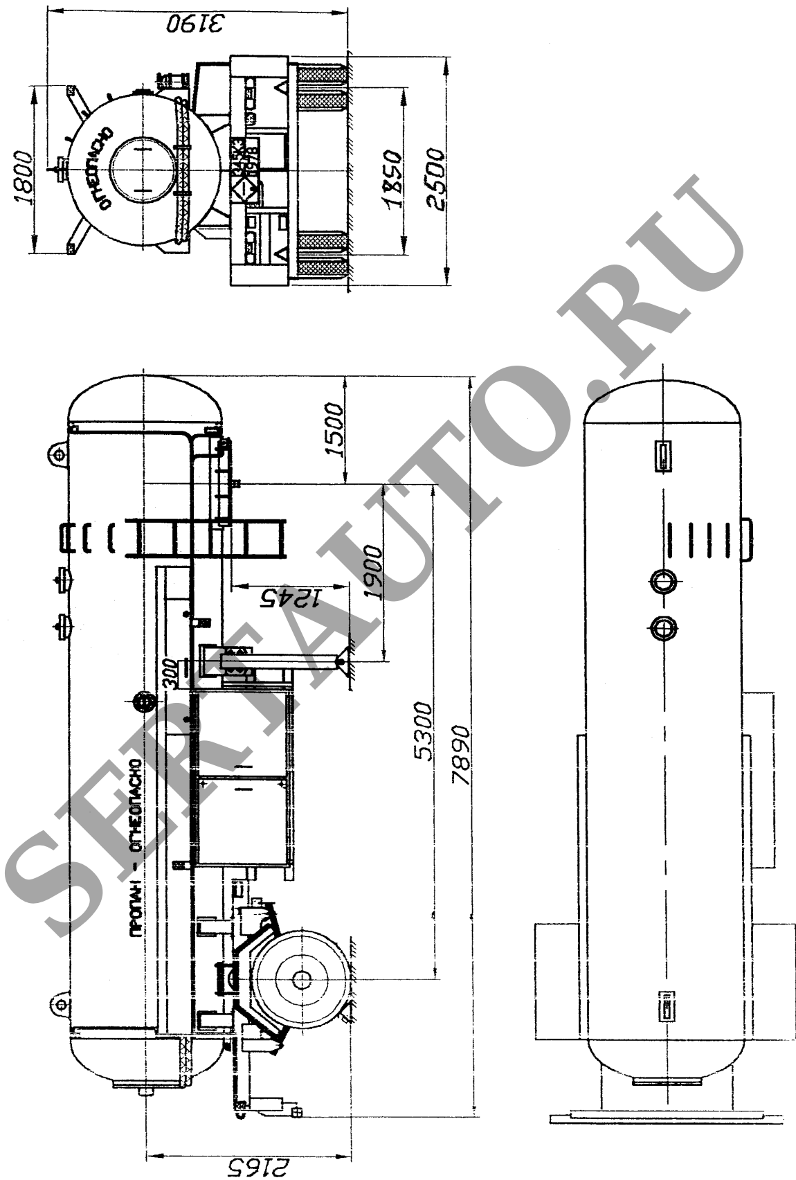
Рис.1. Полуприцеп-топливозаправщик модели 9611TN (9611-000010-01)
