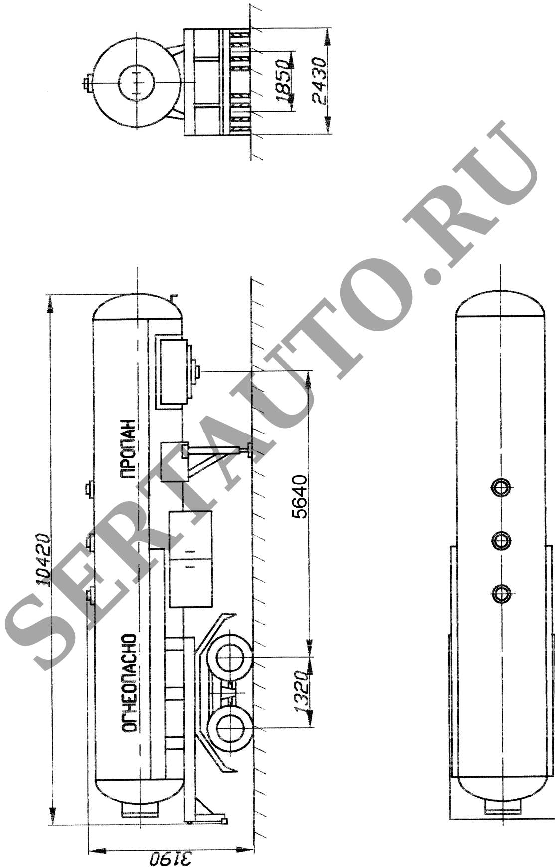
Рис.1. Полуприцеп-цистерна модели 96111 (96111-0000010)
