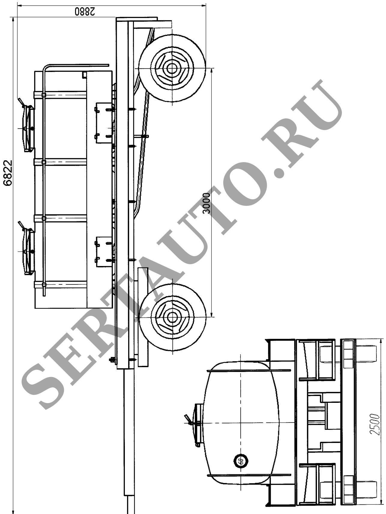
Рис.1. Прицеп-цистерна модели 8620 (8620-0000010) / Г6-ОПА-4,9/3-02
