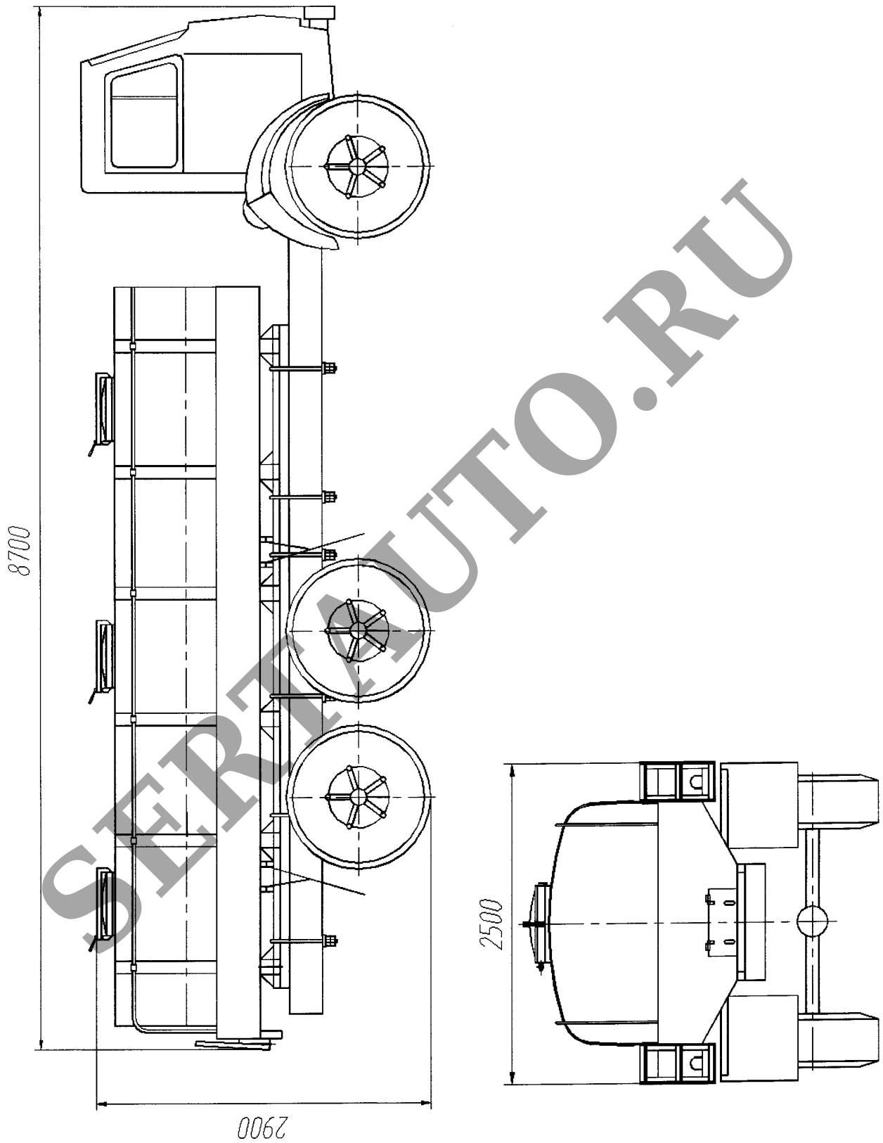
Рис.1. Автоцистерна модели 56581 (5658-000010-10) / (Г6 - ОПА - 4310) на шасси КамАЗ 43118-02
