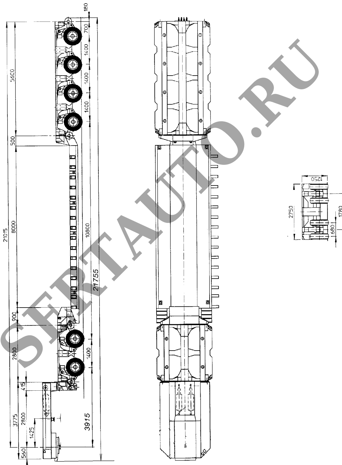
Рис.1. Полуприцеп GOLDHOFER модели STZ - VH6(0+4) / (2+4) TNP/ET.
