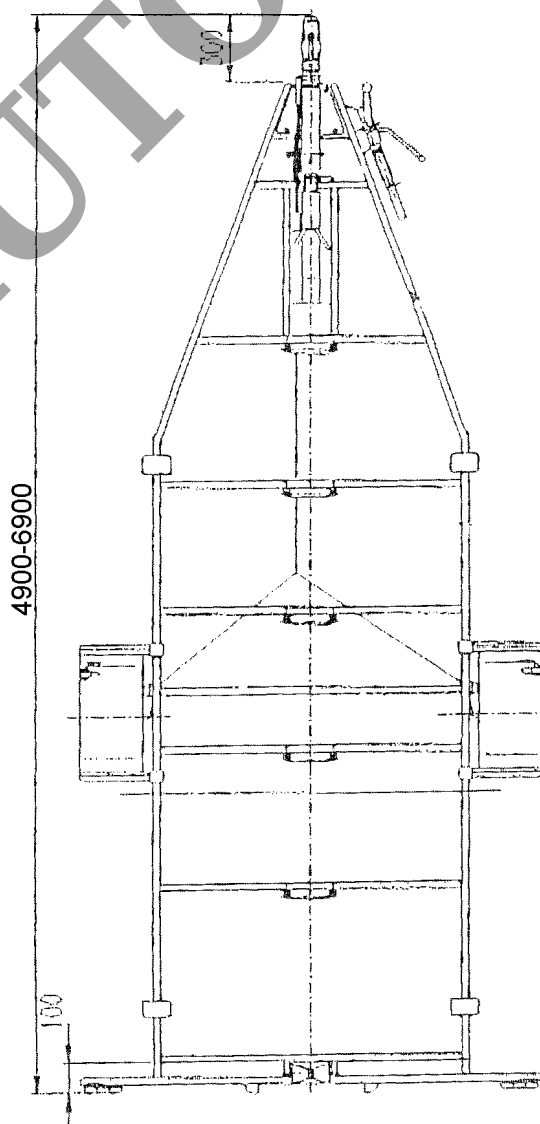
Рис. 1 Прицеп к легковым автомобилям моделей: PC 1000..., PC 1100..., PC 1200..., PC 1500...
